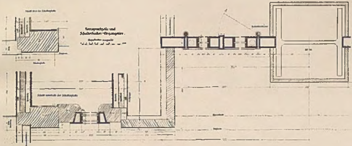
POSTAMT AN DER THERESIENSTRASSE Fernsprechkabine und Schnitt durch die Eingangstüre (Zu Seite 186 oben) i. M. 1:5
