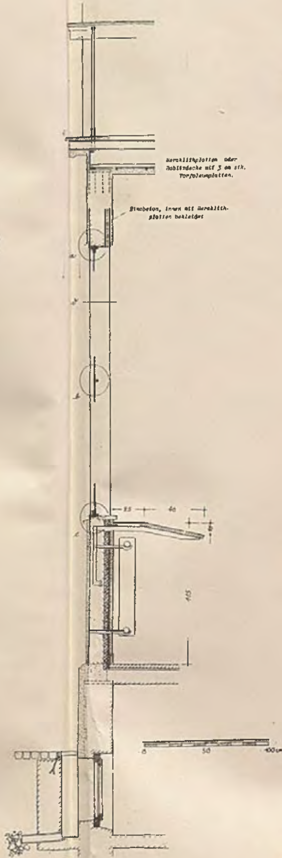
Postamtumbau an der Leopoldstraße Schnitt durch die Konstruktion der Außenfenster. (Zu Seite 176 oben)
