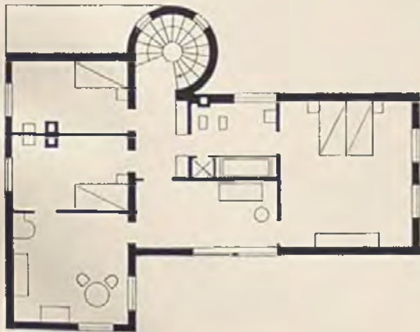
Grundriß Obergeschoß
