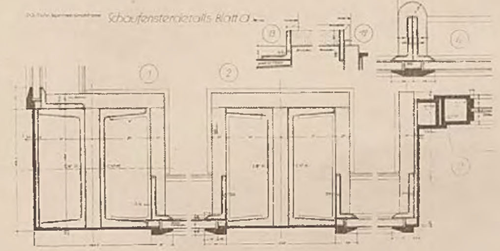
Einzelheiten der Schauenster am Ladenanbau
