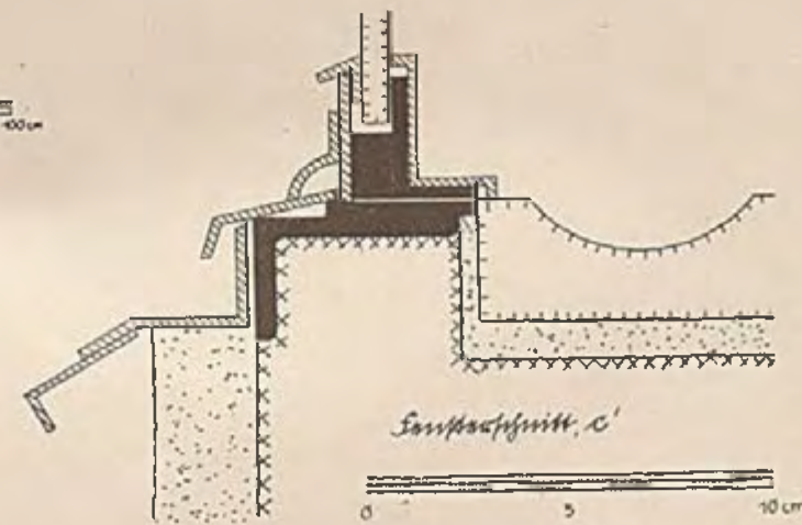
Postamtumbau an der Leopoldstraße Schnitt durch die Konstruktion der Außenfenster. (Zu Seite 176 oben)
